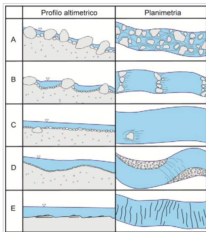
Figura 1.6 – Classificazione dei corsi d'acqua montani secondo MONTGOMERY & BUFFINGTON (1997) . (A) Cascade; (B) a gradinata ( step-pool ); (C) letto piano ( plane bed ); (D) riffle-pool ; (E) dune-ripple .
